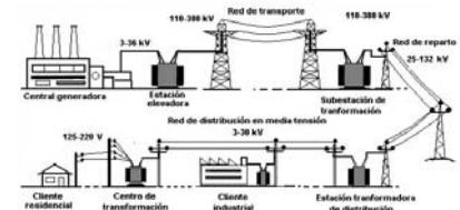
*Esquema de transmisión de energía por Redes primarias
